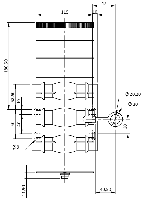
Anschluss C (Steckverbinder M16, 8-polig DIN)
