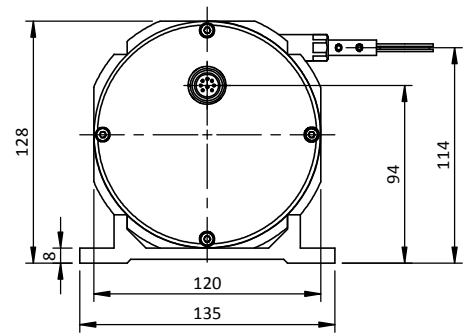
Anschluss C (Steckverbinder M16, 8-polig DIN)
