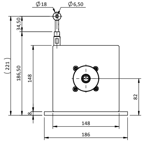
Connectique C (Connecteur M16 - DIN 3 broches)
