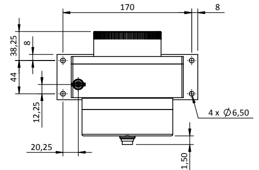
Connectique C (Connecteur M16 - DIN 3 broches)
