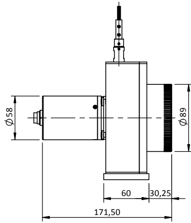
Connectique L4 (connecteur M12 - 4 broches)
