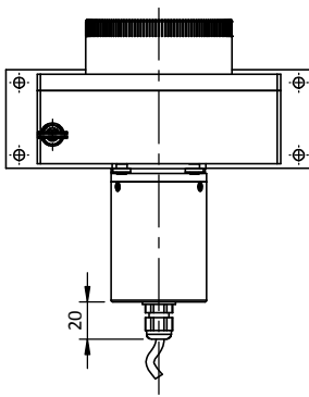
Connectique K (Câble PVC - 4 fils)
