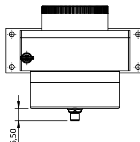
Connectique L4 (connecteur M12 - 4 broches)
