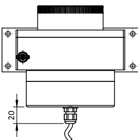
Connectique K (Câble PVC - 4 fils)
