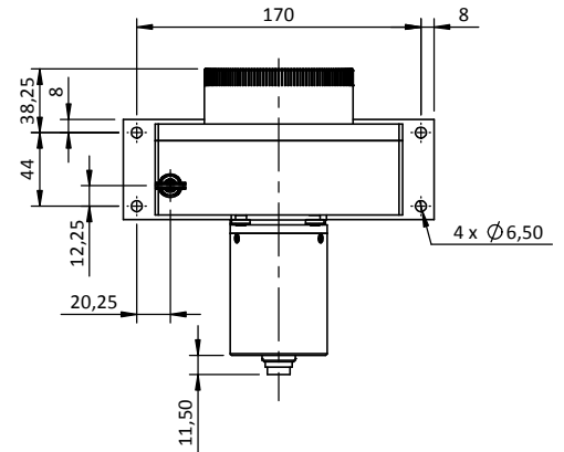
Connectique C (Connecteur M16 - DIN 3 broches)
