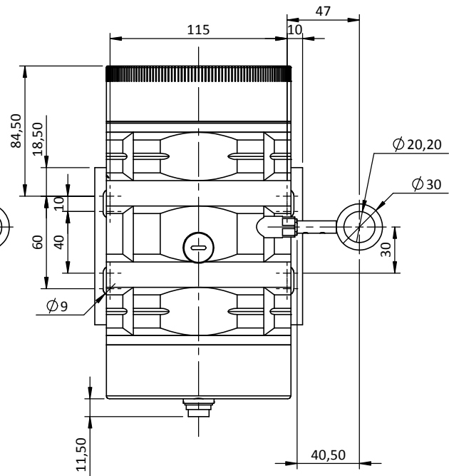
Connectique C (connecteur M16 - DIN 3 broches)
