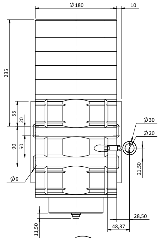
Connectique C (Connecteur M16 - DIN 3 broches)
