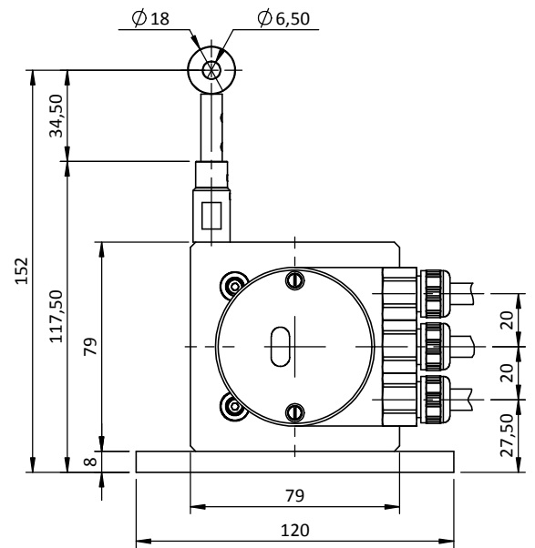
Codeur MHM5 - PROF/CANO/DNET Connectique H3P ou OCC (Boîte à bornes)
