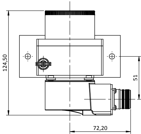
Codeur PHM5 - SSI Connectique S6R ou S8R (Connecteur mâle M23 - 12 broches sens horaire ou anti-horaire)
