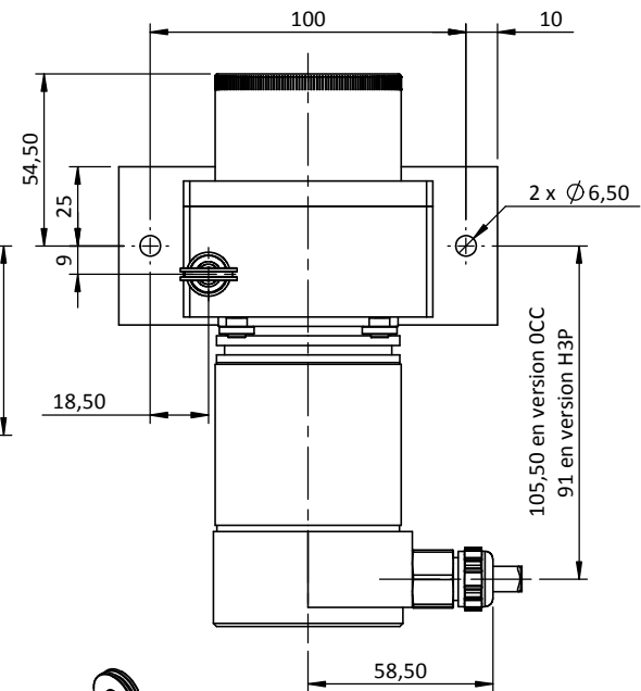
Codeur MHM5 - PROF/CANO/DNET Connectique H3P ou OCC (Boîte à bornes)
