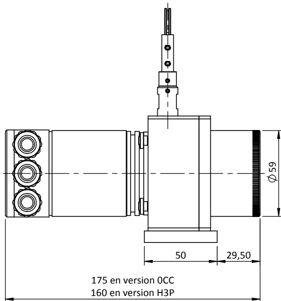
Codeur PHM5 - SSI Connectique S6R ou S8R (Connecteur mâle M23 - 12 broches sens horaire ou anti-horaire)
