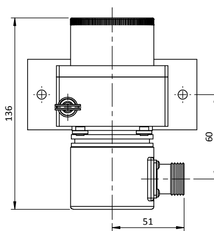
codeur MHM5 - SSI Connectique PRL (Connecteur mâle connector M23 - 12 broches sens anti-horaire)
