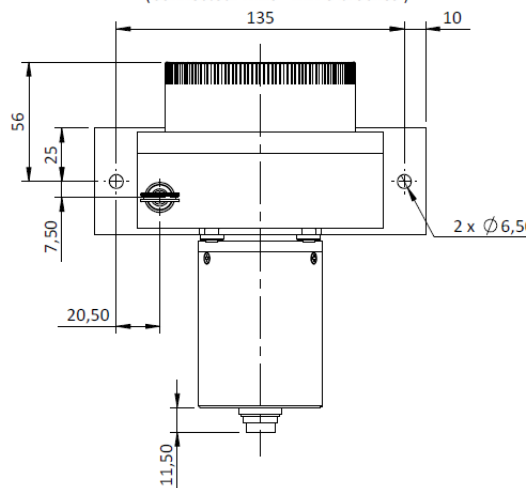
Connectique C (Connecteur M16 - DIN 8 broches)
