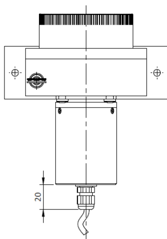
Connectique K (Câble PVC - 4 fils)
