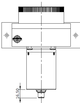
Connectique L4 (connecteur M12 - 4 broches)
