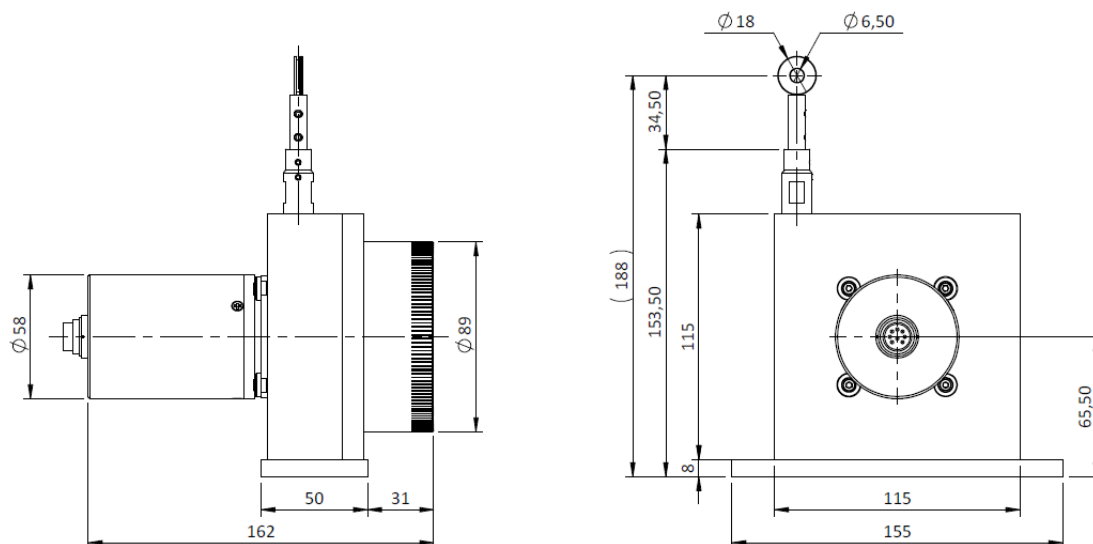
Connectique K (Câble PVC - 4 fils)
