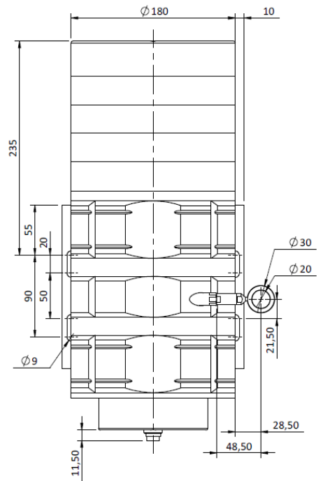
Connectique C (Connecteur M16 - DIN 8 broches)
