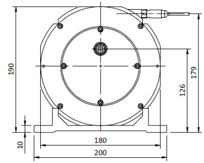
Connectique C (Connecteur M16 - DIN 8 broches)
